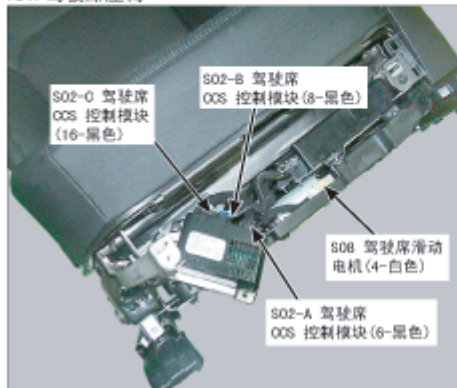
151. 驾驶席座椅
