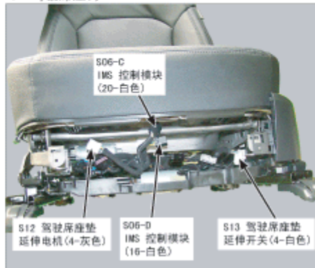
152. 驾驶席座椅
