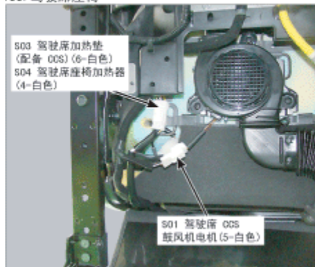
155. 驾驶席座椅
