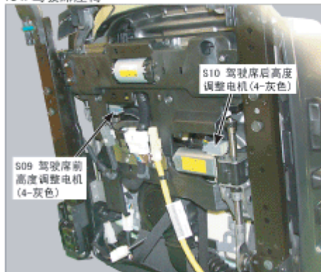
154. 驾驶席座椅
